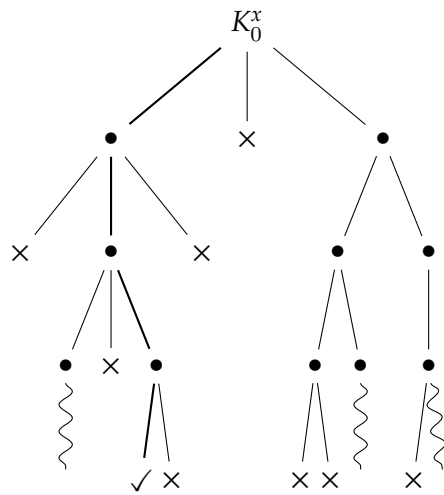
Strom nedeterministického výpočtu
